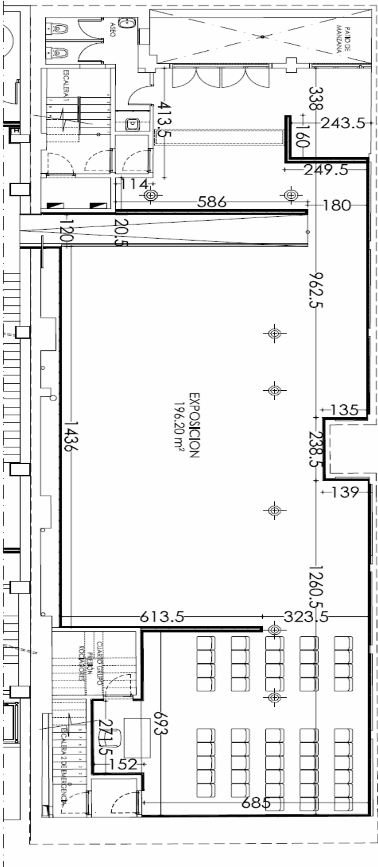
PLANTA SOTANO Esc.: 1/100
